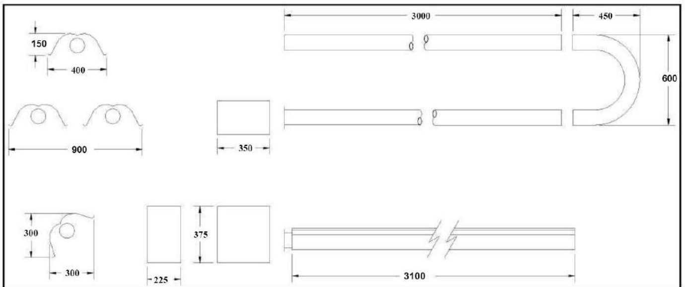
Рисунок 1 наружные размеры частей оборудования
